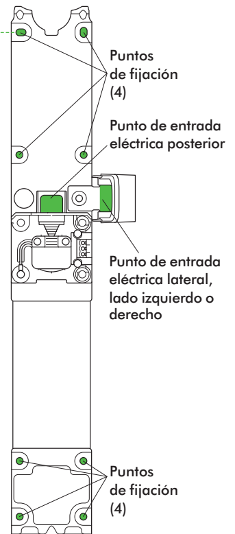
PLACA TRASERA
