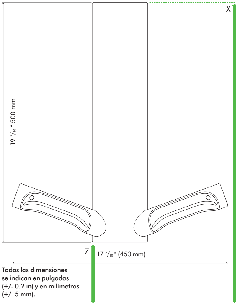
ELEVACIÓN FRONTAL
